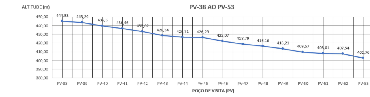
PERFIL DE ELEVAÇÃO: PV-38 AO PV - 53
