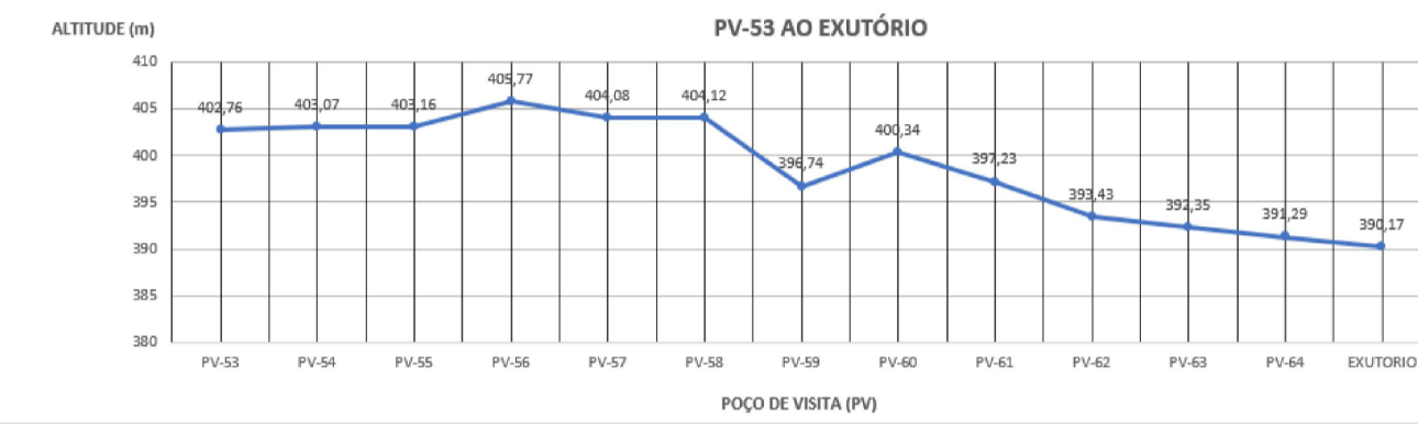
PERFIL DE ELEVAÇÃO: PV - 53 AO EXUTÓRIO
