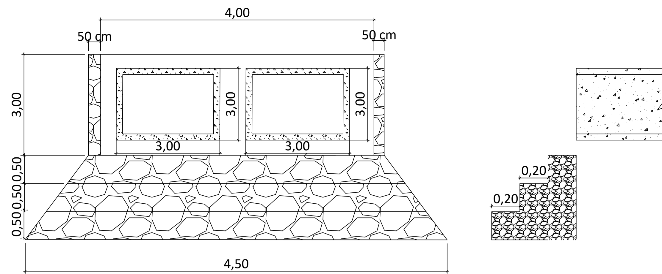
07 DETALHE DISSIPADOR DE ENERGIA ESC.: 5/ESC
