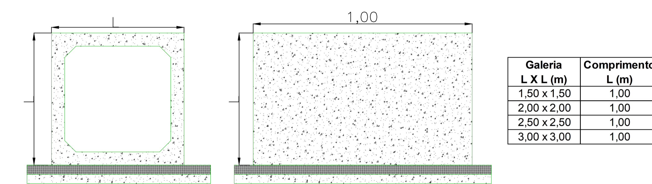
08 DETALHE GALERIA QUADRADA / TUBO ESC.: 5/ESC
