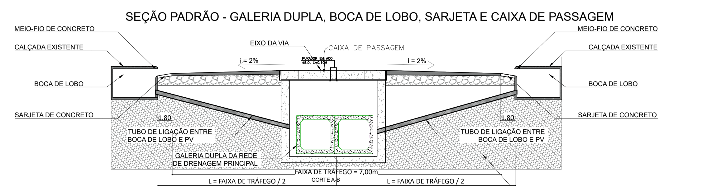
06 SEÇÃO TRANSVERSAL - PADRÃO 10 ESC.: 1/50
