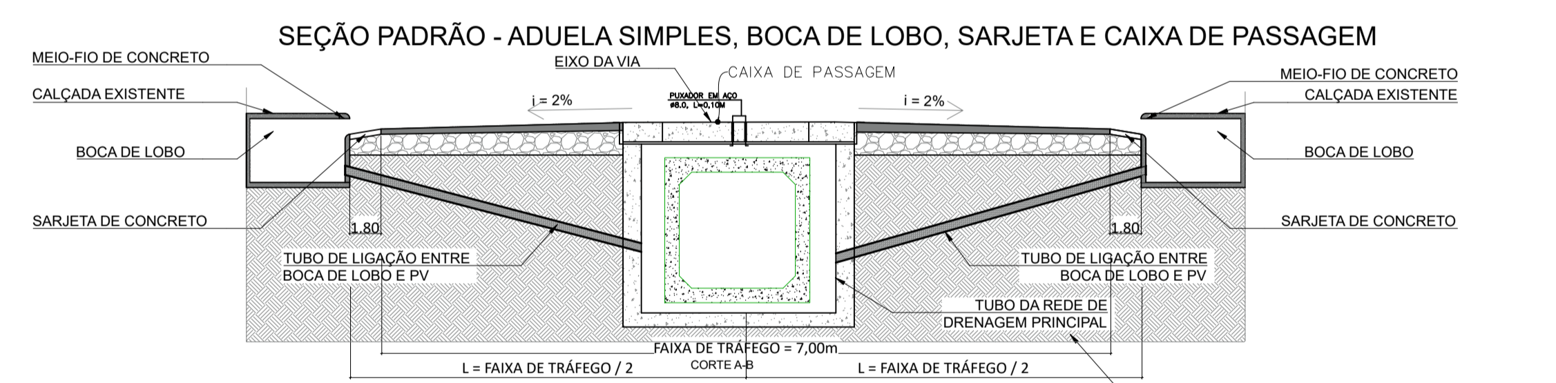
04 SEÇÃO TRANSVERSAL - PADRÃO 06 ESC.: 1/50
