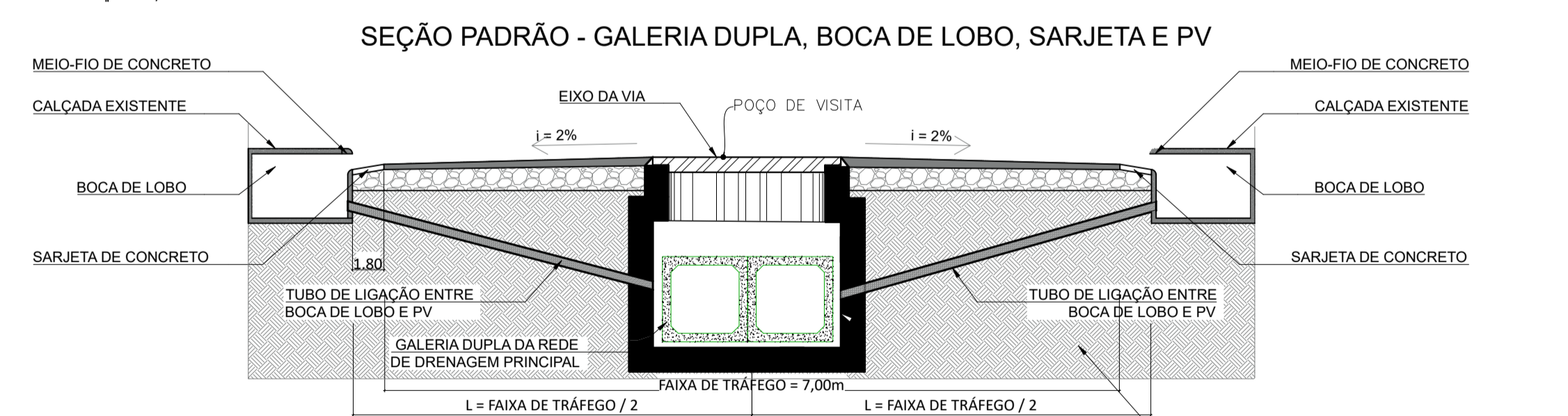
05 SEÇÃO TRANSVERSAL - PADRÃO 09 ESC.: 1/50
