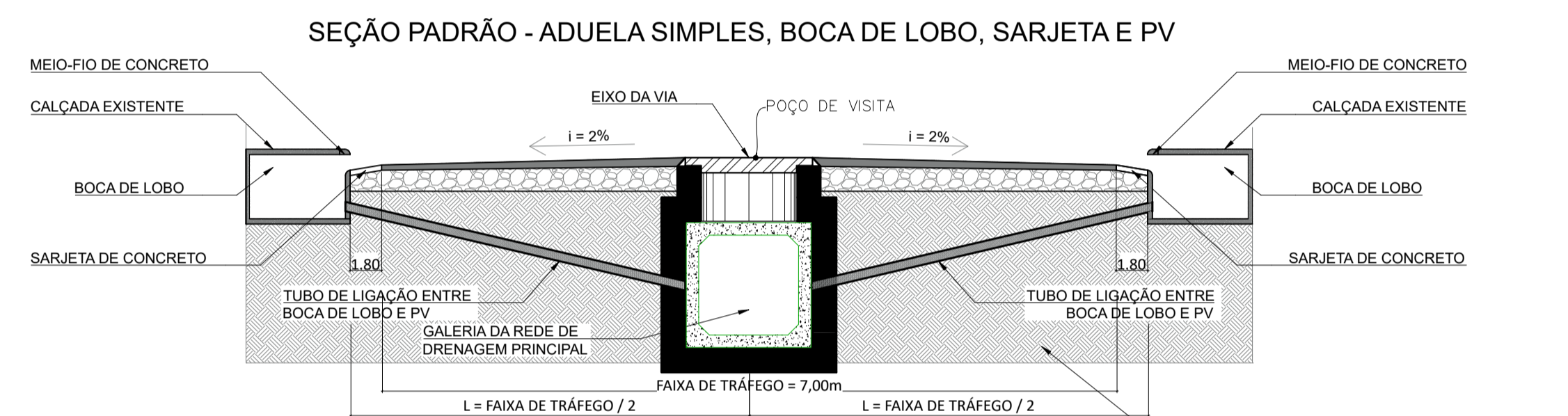
03 SEÇÃO TRANSVERSAL - PADRÃO 05 ESC.: 1/50
