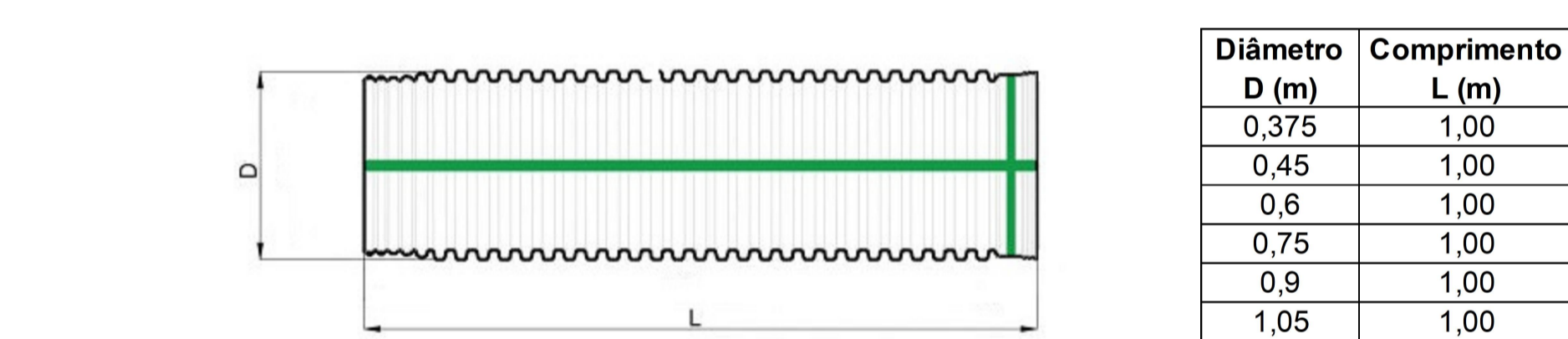
09 DETALHE TUBO PEAD ESC.: 5/ESC
