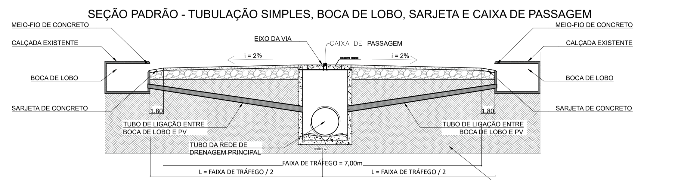
02 SEÇÃO TRANSVERSAL - PADRÃO 02 ESC.: 1/50
