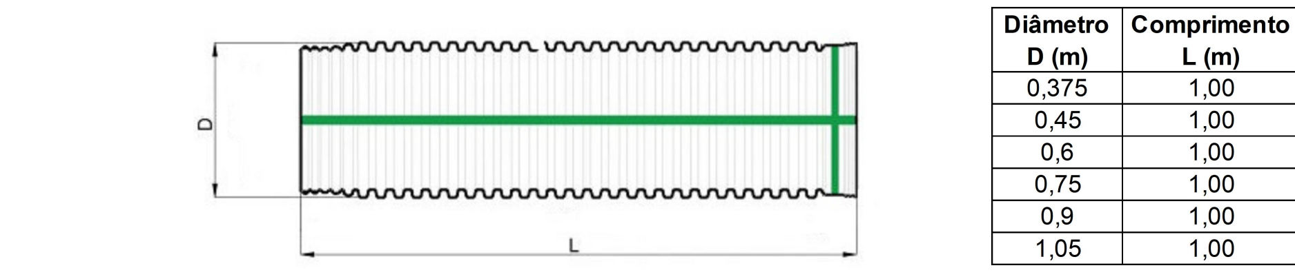
07 DETALHE TUBO PEAD ESC.: S/ESC
