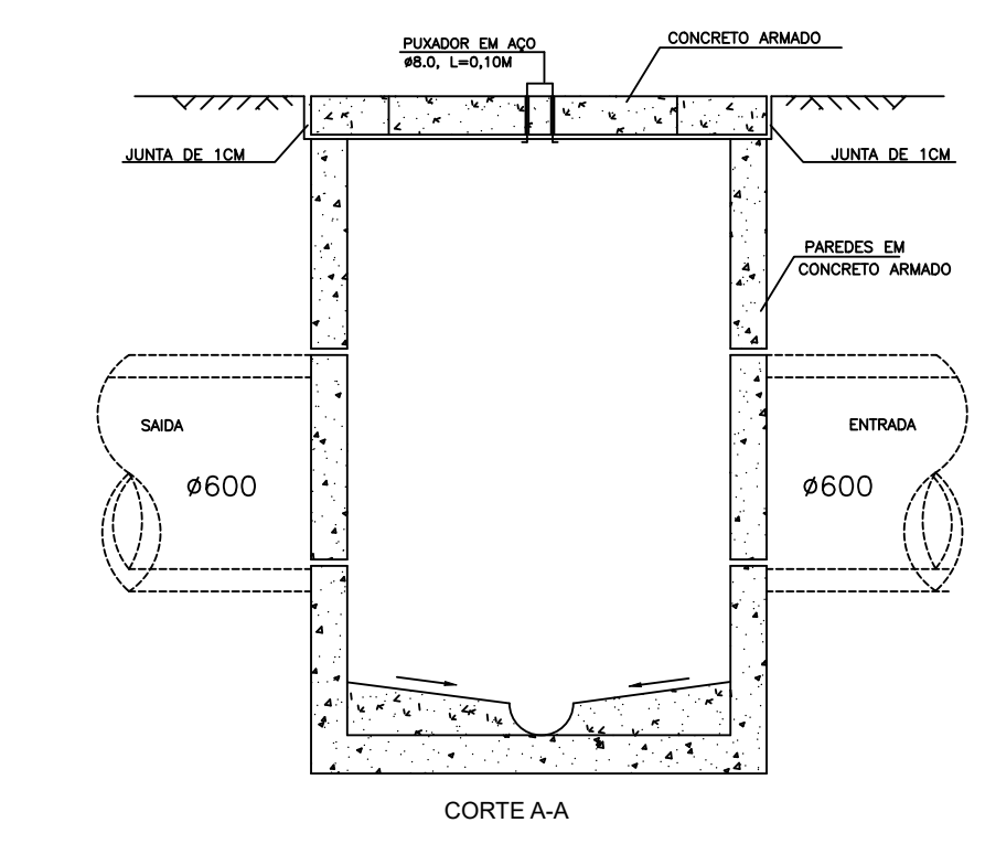
09 DETALHE CAIXA DE PASSAGEM ESC.: S/ESC
