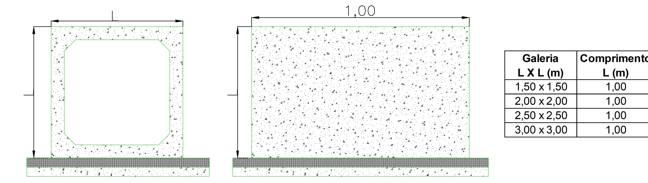
06 DETALHE GALERIA QUADRADA / TUBO ESC.: S/ESC
