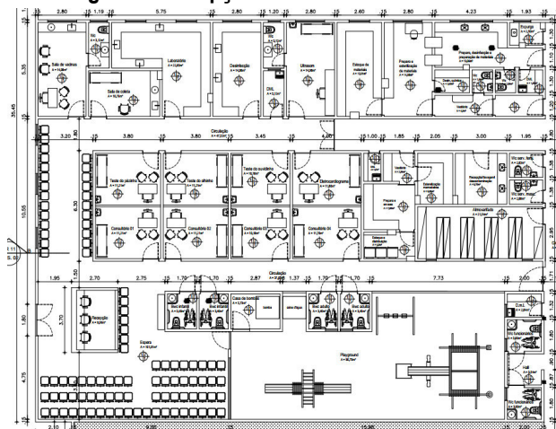
Figura 4. Recepção da Unidade Ambulatorial
