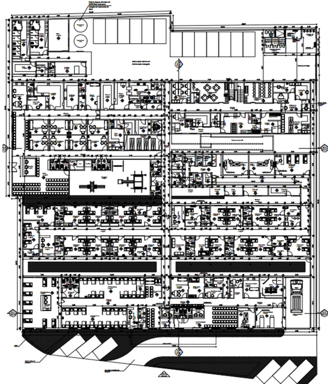
Figura 2 – Planta Baixa do Térreo do Hospital Infantil Maria Amélia (HIMA)
