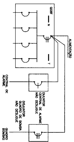
DIAGRAMA ALIMENTAÇÃO BOMBA INCÊNDIO/ CENTRAL SEM ESCOVA
