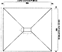
SSZ CORTA ESC: 1/25
