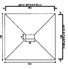
S15 PLANTA ESC: 1/20
