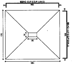
S4=S35 PLANTA ESC. 1:20
