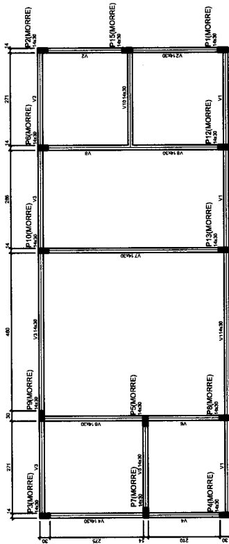
Forma do pavimento TÊRREO escala: 1:50
