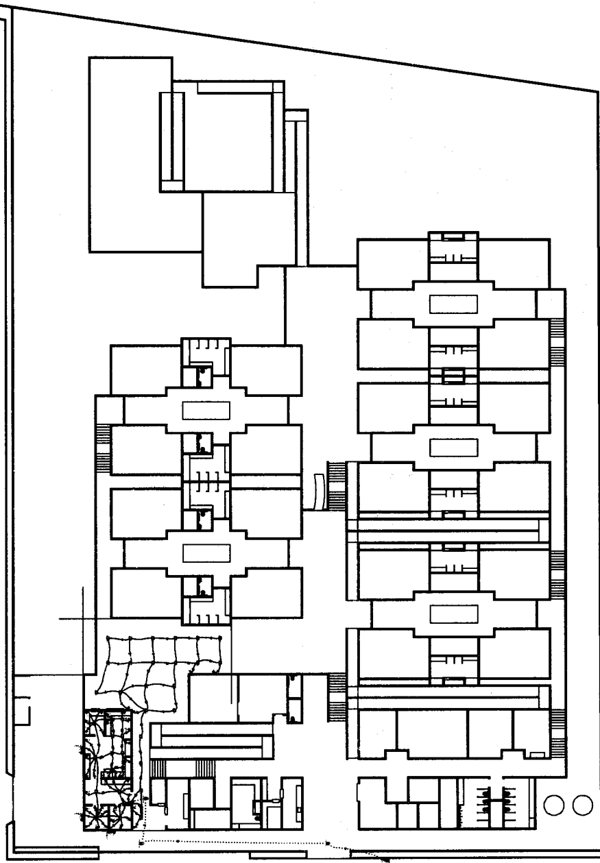
PLANTA BAIXA ESCALA 1/200
