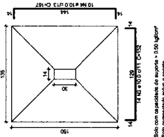
S23=SS2 PLANTA ESC 1:25
