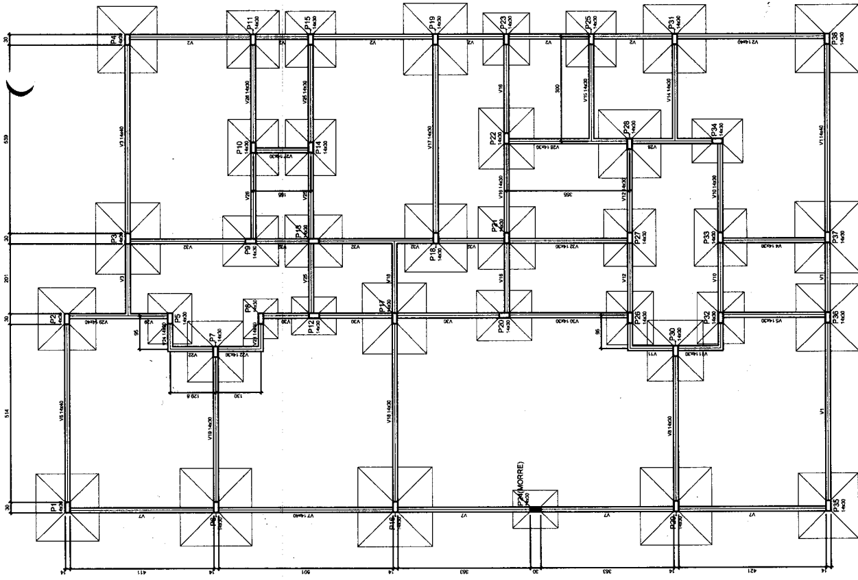
Forma do pavimento Baldrame
