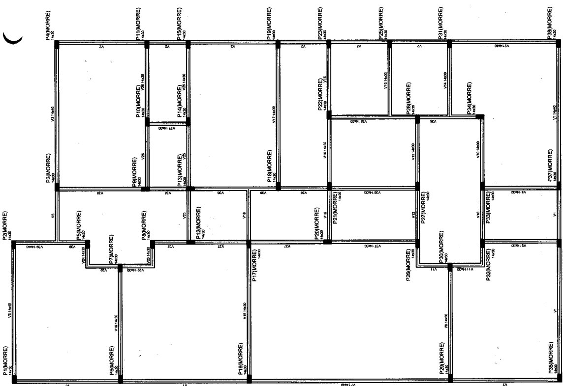
Forma do pavimento terreo escala 1:50
