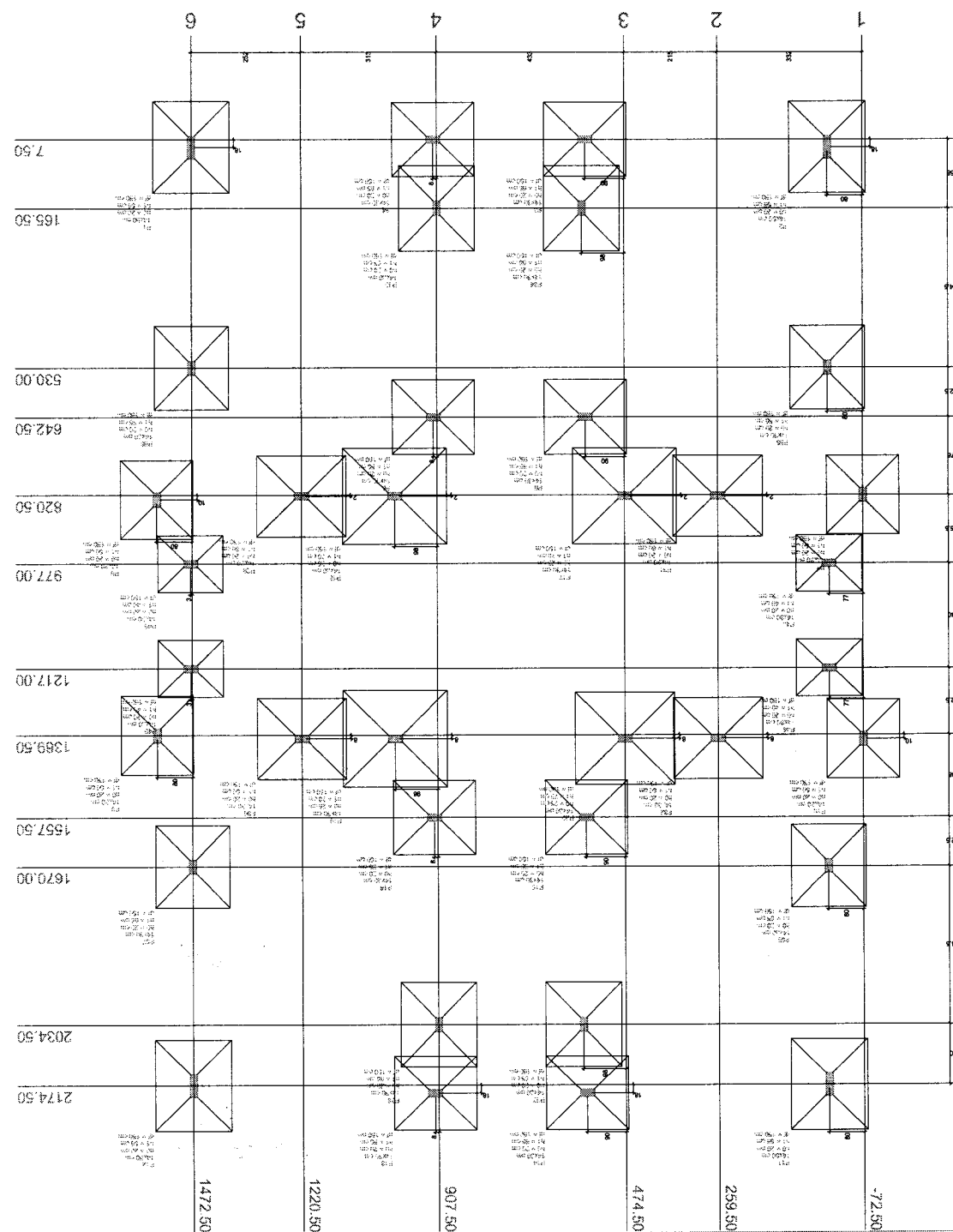
Planta de locação
