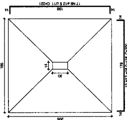
S3=S17=S19=S37 PLANTA ESC. 1:20
