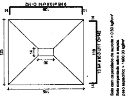
S4=S34 PLANTA ESC. 1:20
