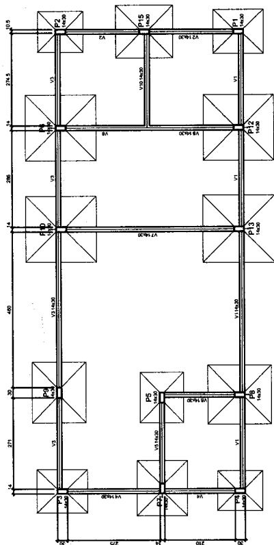
Forma do pavimento BALDRAME escala: 1:50
