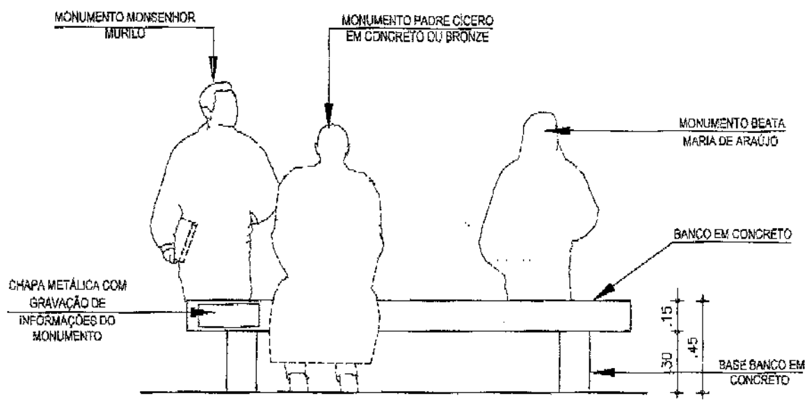
02 VISTA 01 ESC. 1/25
