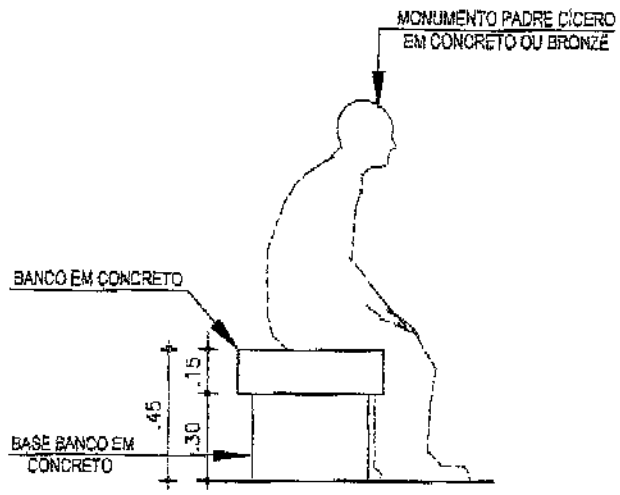
03 VISTA 02 ESC. 1/25
